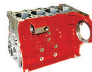
Блок цилиндров в сборе 5261256/5261257
