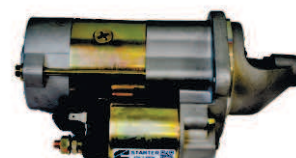
Стартер 12V 2,5kW 5266969/5311304/5295576
