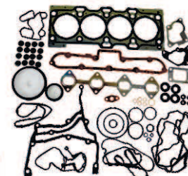
Комплект прокладок двигателя DP05651195
