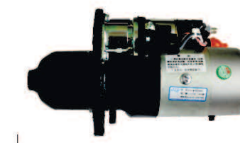
Стартеры 5263797-Валдай, 5268413/5263841/5319202-ПАЗ
