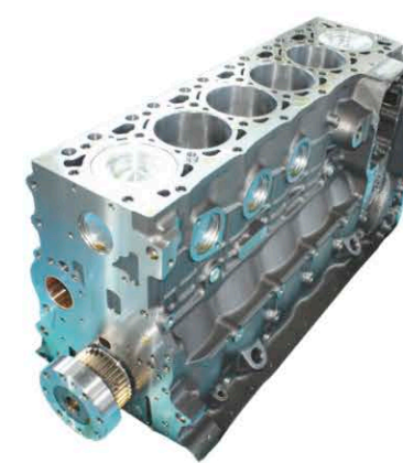
Сервисный двигатель 6ISBe (EURO3) третьей комплектности (short block) SO75250
