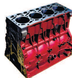
Блок цилиндров 5289698/5306413-Евро 3 5289699/5306414-Евро 4
