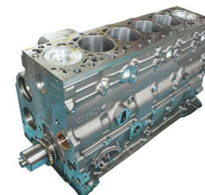
Сервисный двигатель 6ISBe6.7 (EURO4) третьей комплектности (short block) SO75340
