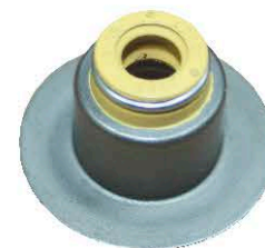
Колпачок маслосъемный ISF3.8, ISBe 4991571/ 3955393
